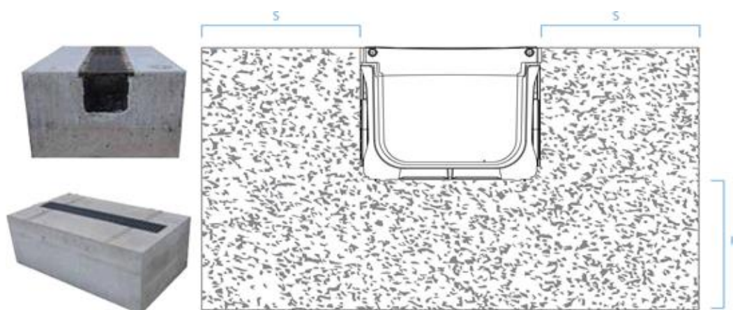
ΠΙΝΑΚΑΣ ΔΙΑΣΤΑΣΕΩΝ ΕΓΚΙΒΩΤΙΣΜΟΥ ΚΑΝΑΛΙΩΝ ΑΝΑ ΚΑΤΗΓΟΡΙΑ ΦΟΡΤΙΣΗΣ
