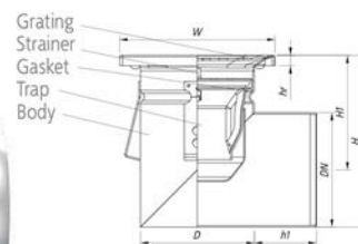
Έξοδος Φ110
