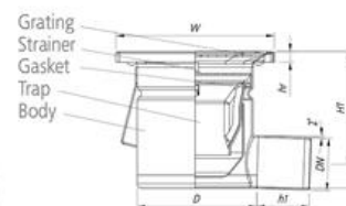
Έξοδος Φ50
