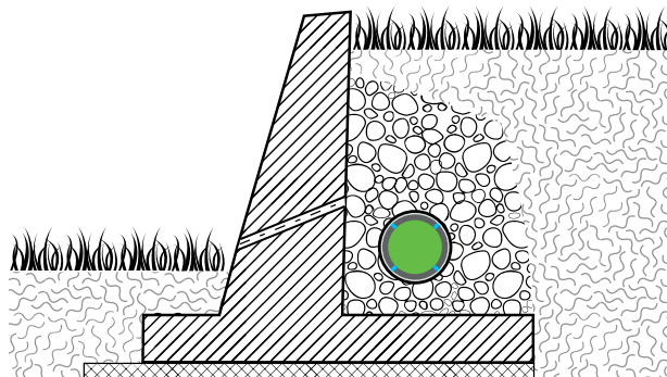
Αποστράγγιση σε τοιχεία οπλισμένου σκυροδέματος
